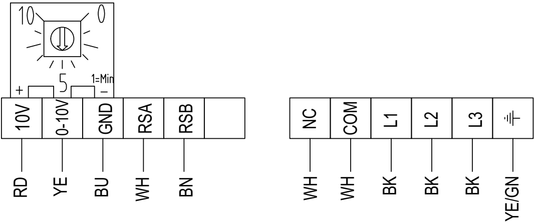
Fig. 5 Revolution 400 EC 3~
