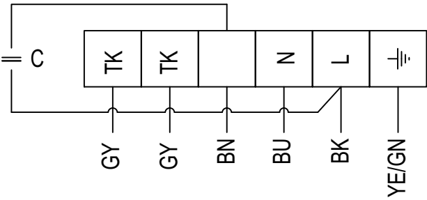
Fig. 3 Revolution 315-400
