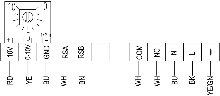
Fig. 4 Revolution 315-400 EC
